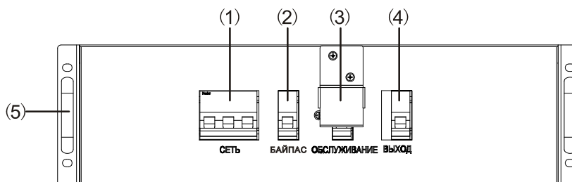
Вид спереди
